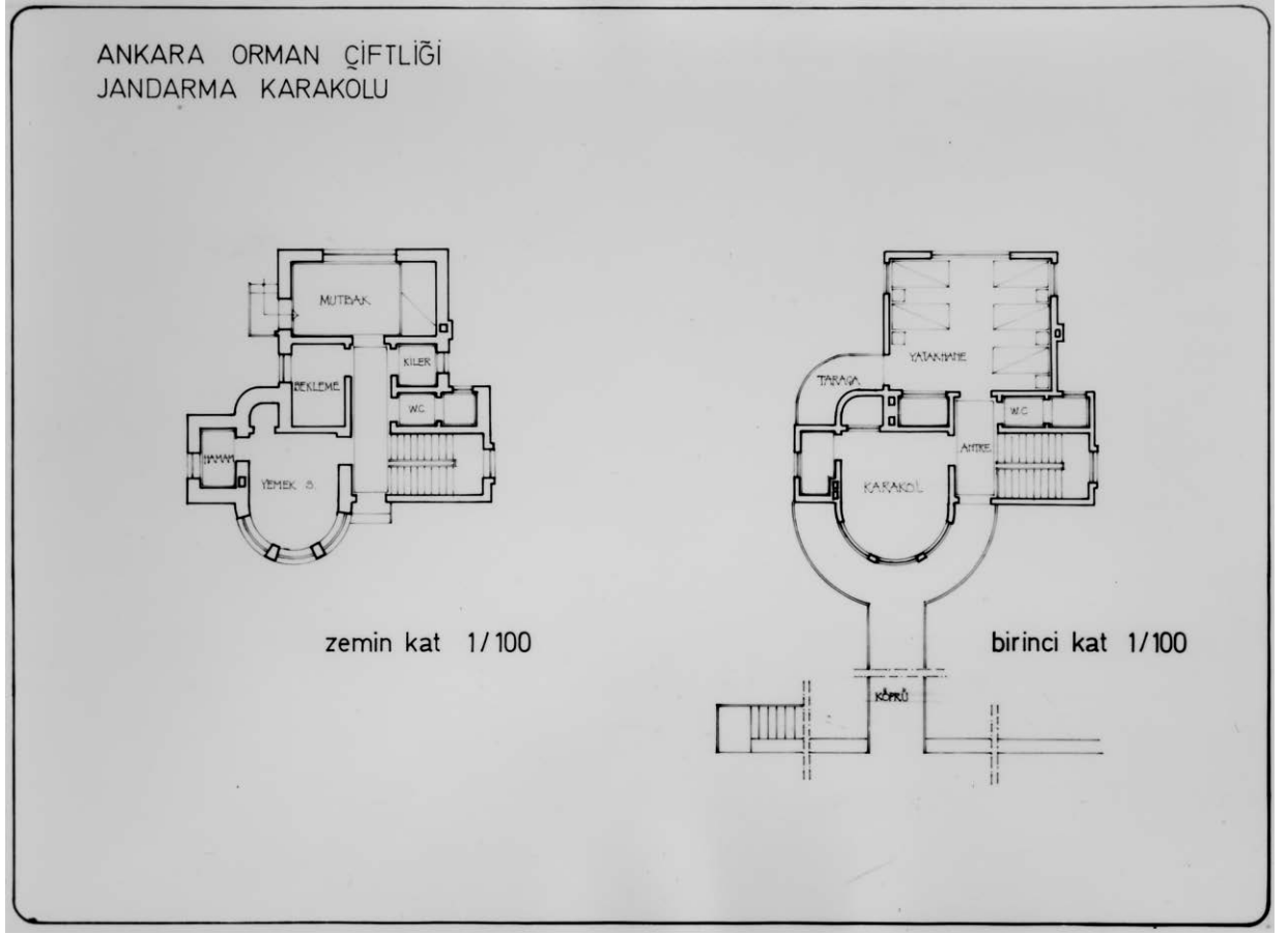
Orman Çiftliği Jandarma Karakolu kat planları (Kaynak: TMMOB Mimarlar Odası Ankara Şubesi Arşivi)
